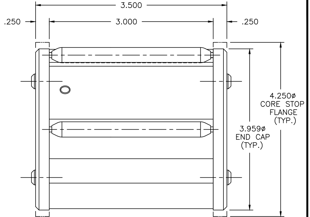
LEFT SIDE
